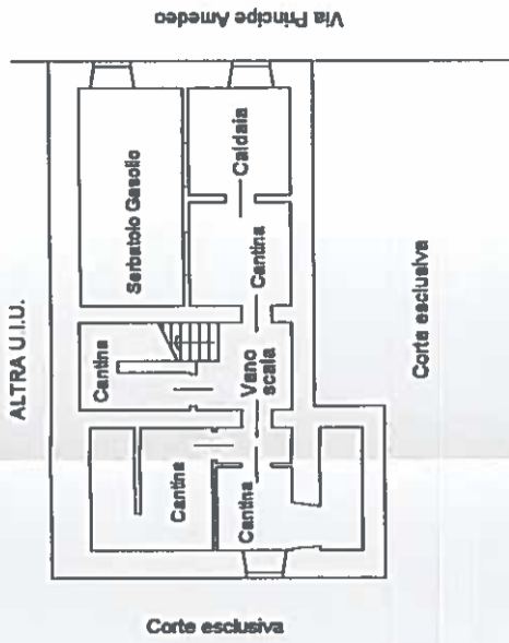
PIANO PRIMO INTERRATO - H 2.50
