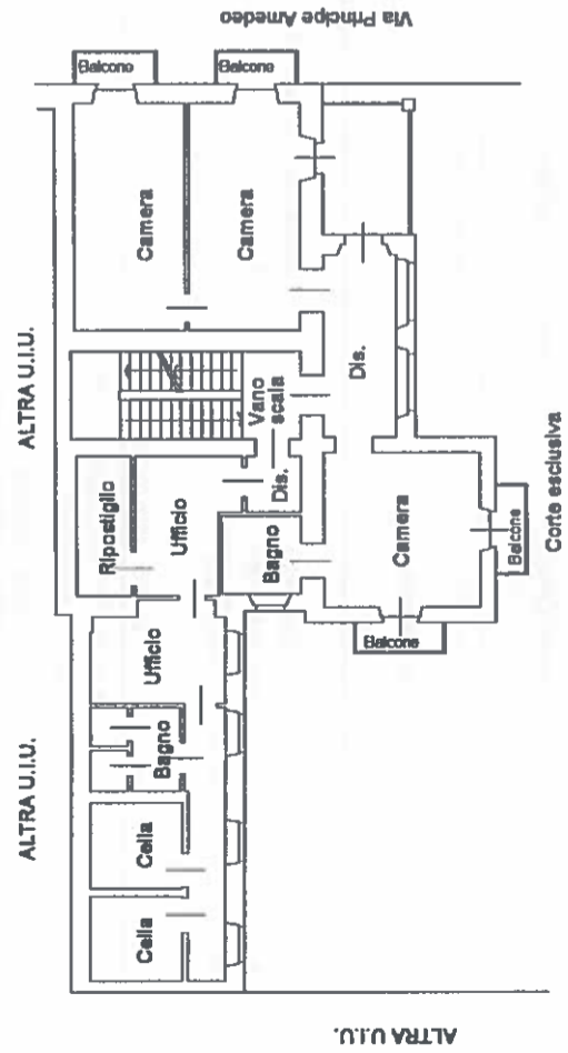
PIANO PRIMO - H 3.30
