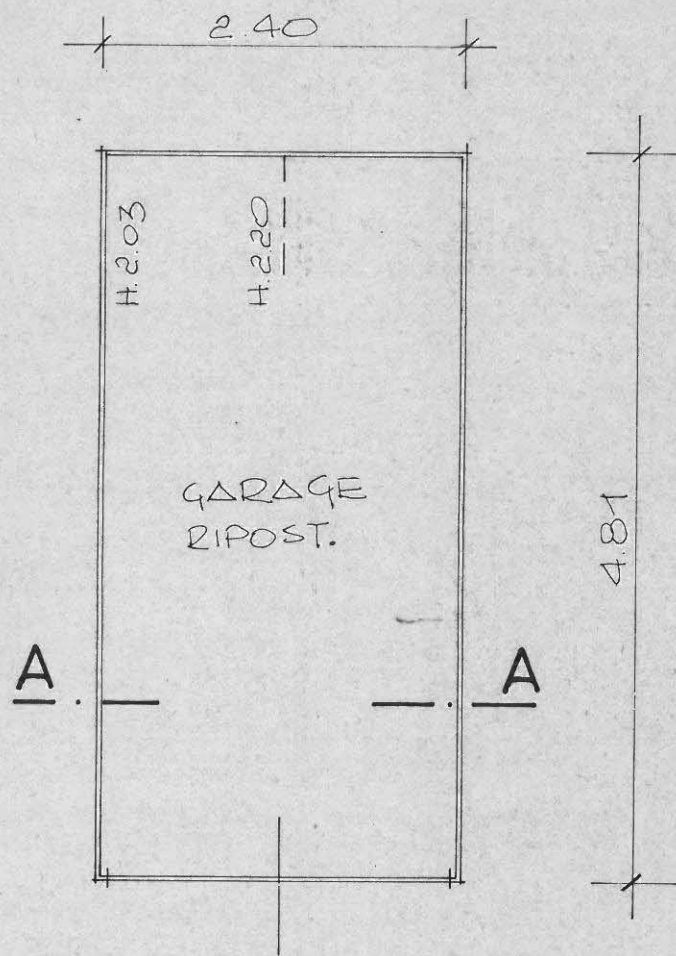
PIANTA 1:50
