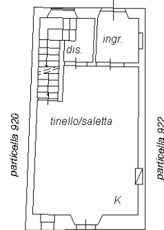
affaccio su particella 931 PIANO TERRA H=2,80
