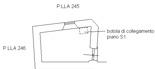
ALTRA U.I. PIANTA PIANO TERRA h. 2,57
