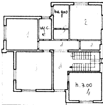
Piano 1°
